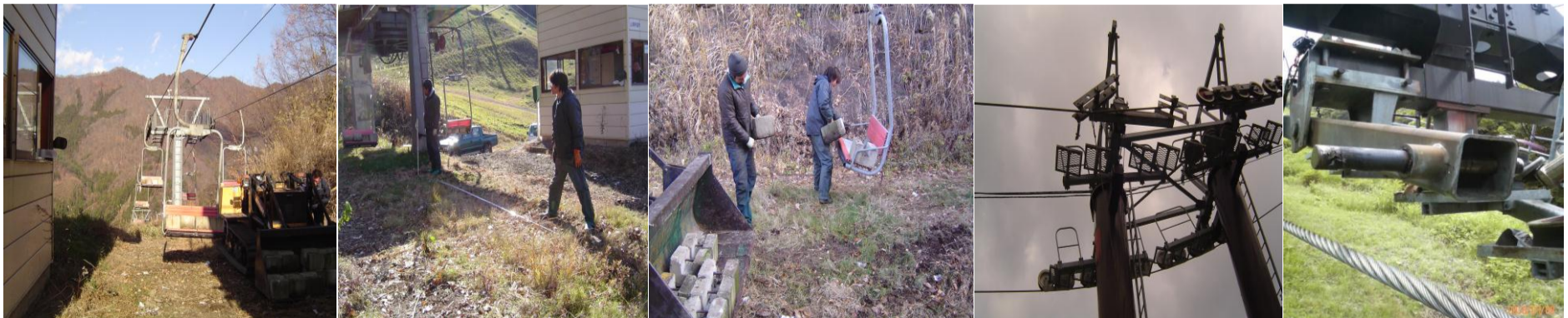
荷重試験風景
